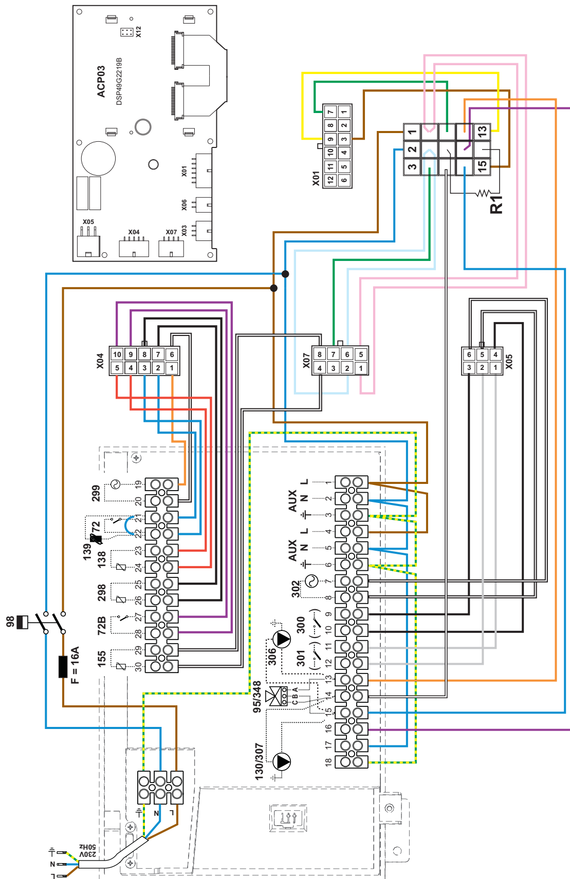
fig. 121- Display wiring diagram
