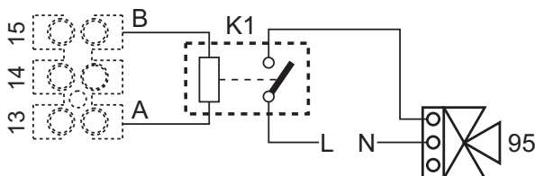
fig. 118 - Collegamento della valvola a 3 vie con 2 fili
