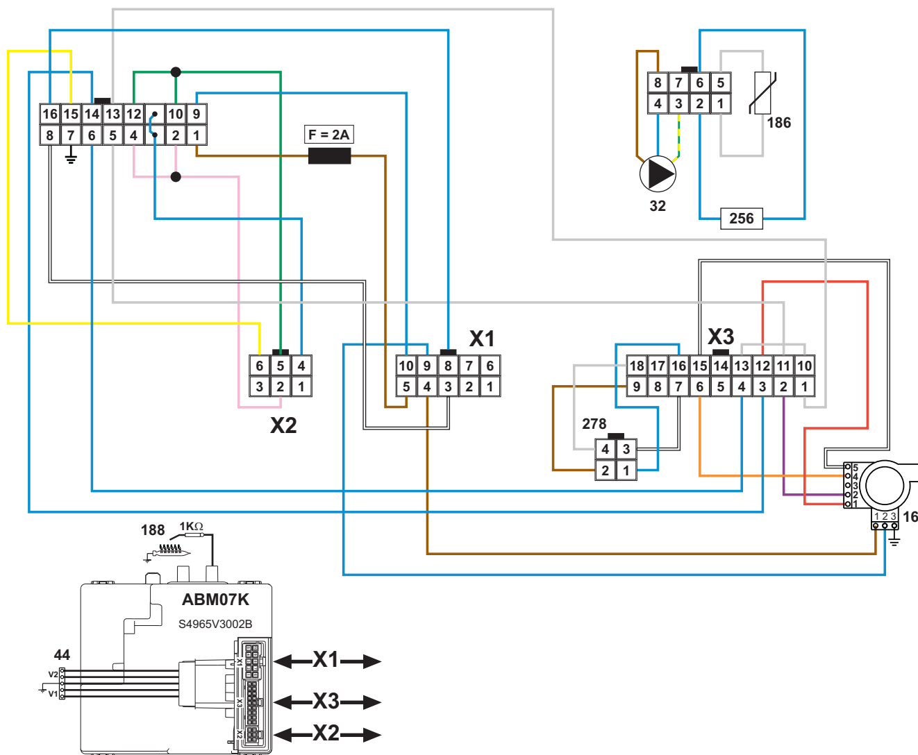
fig. 124- Last module wiring diagram
