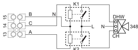
fig. 119 - Collegamento della valvola a 3 vie con 3 fili
