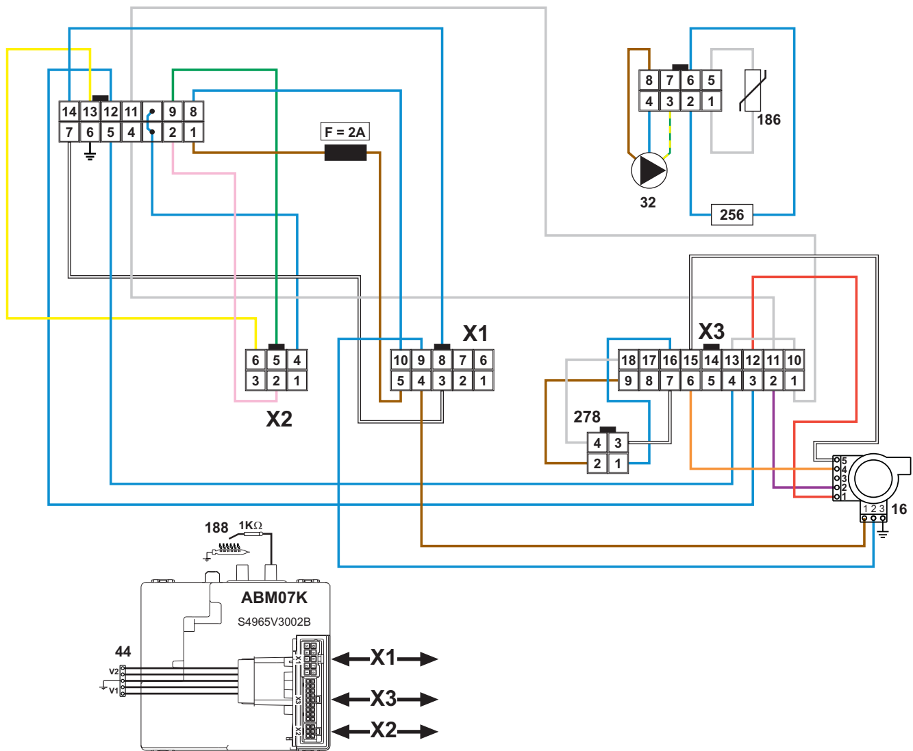
fig. 123 - Schema elettrico Modulo intermedio
