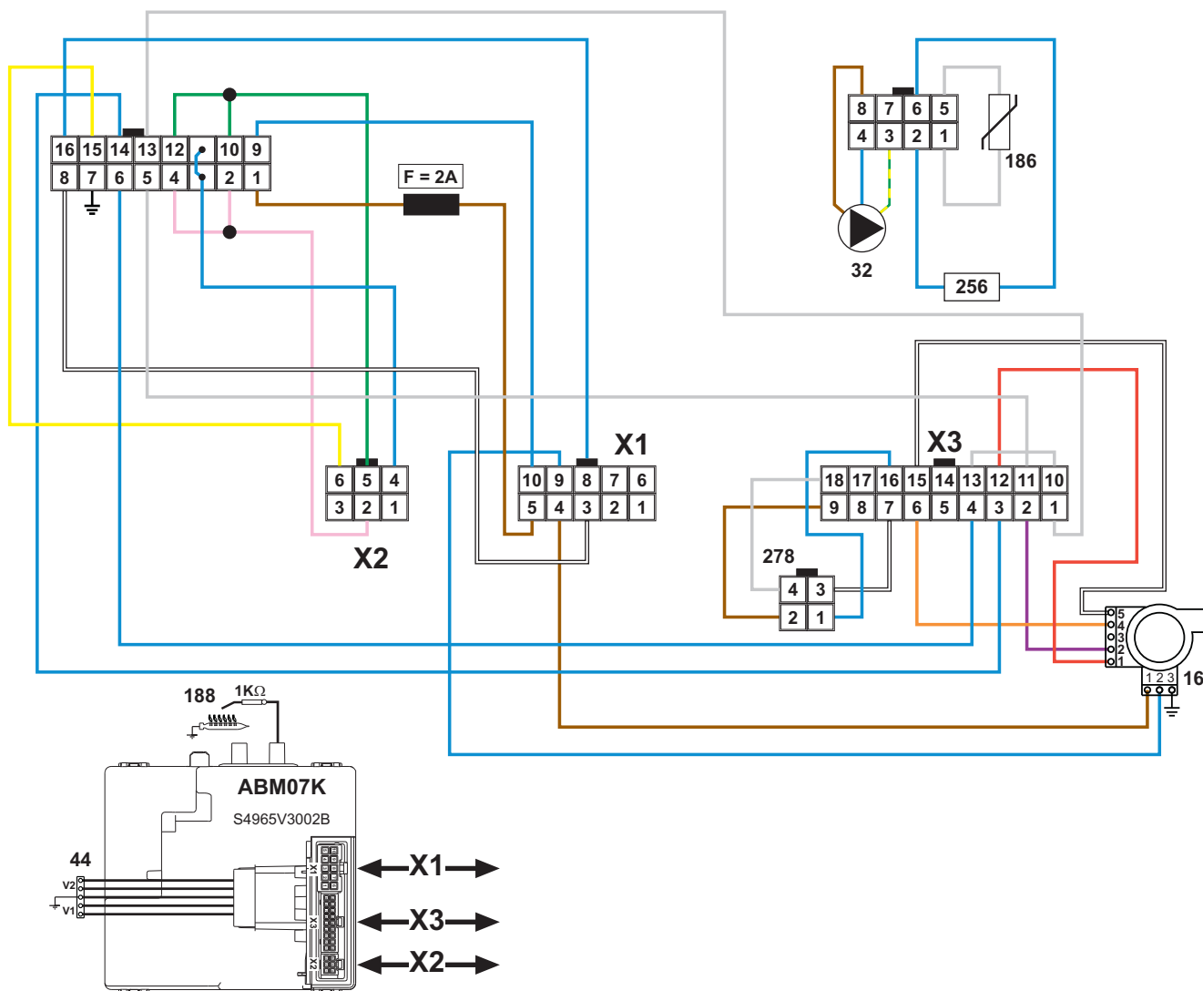
fig. 124 - Schema elettrico Ultimo modulo
