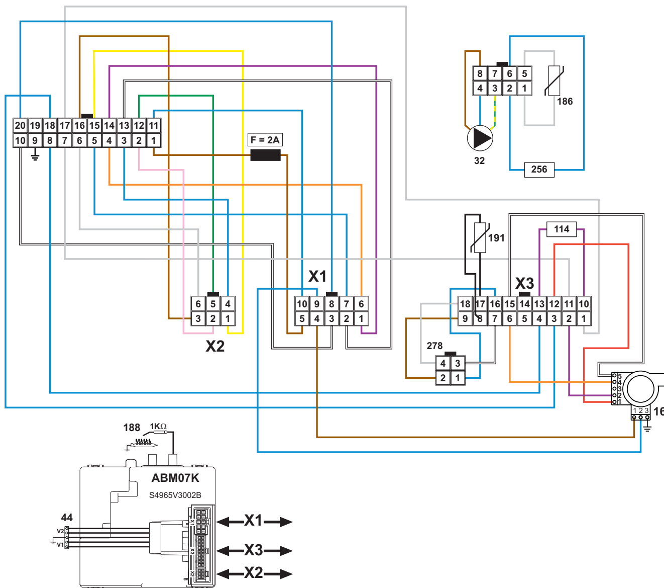
fig. 122 - Schema elettrico Primo modulo
